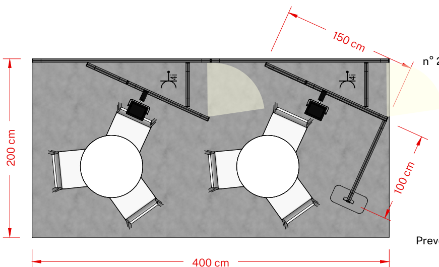
pianta | plan *
