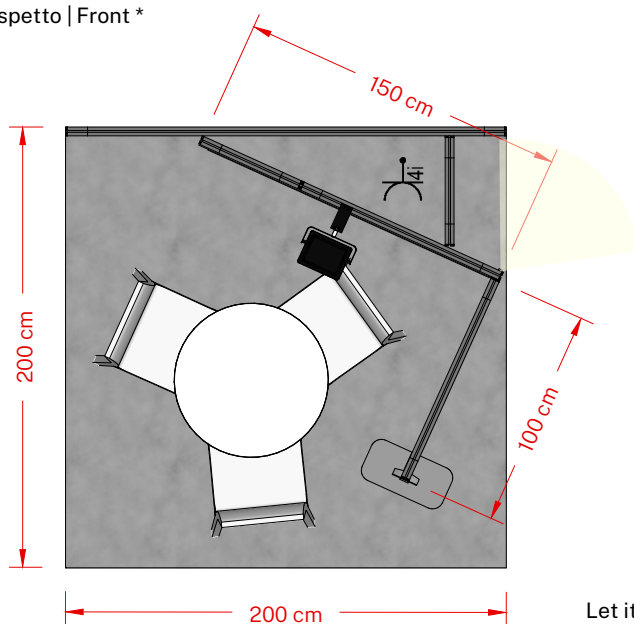
pianta | plan *
